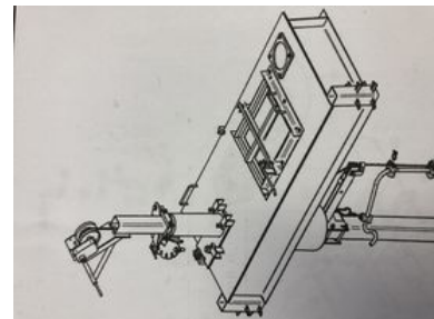
Servisný otvor s uchytením žeriavu
