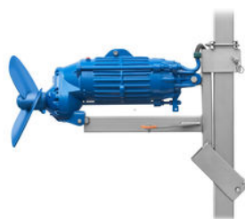
Miešadlo s ponorným motorom EISELE GTWSI 1040
