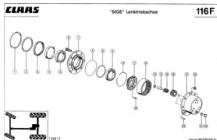
Opatrebitel'ny kruh
